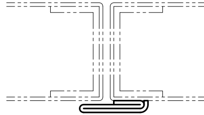
納まり参考図 1:1
