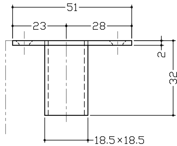
5400-1B 330用先金ガイド (5400-330のみ 使用可)
