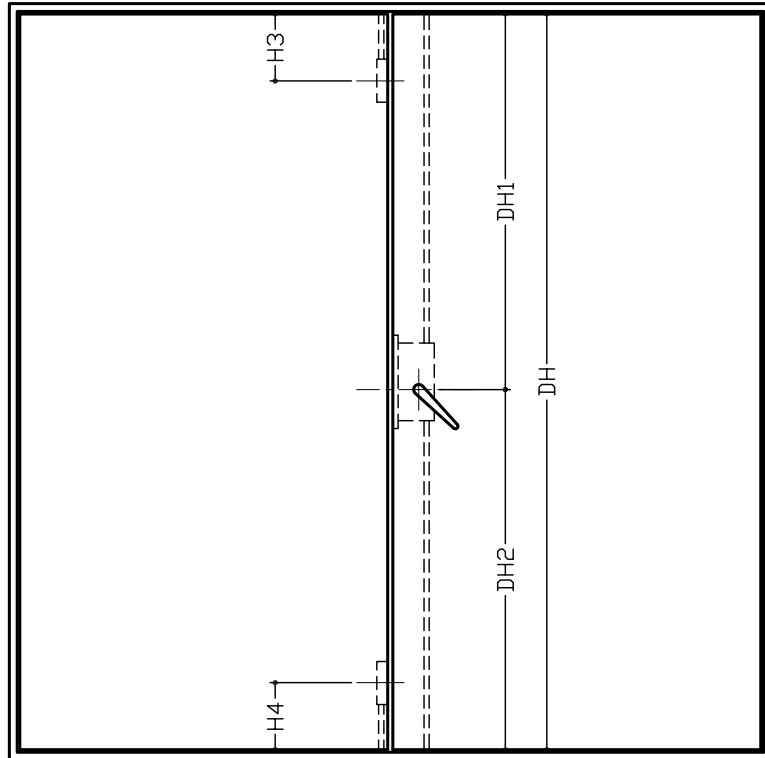
グレモン錠・ロッド 関係図
