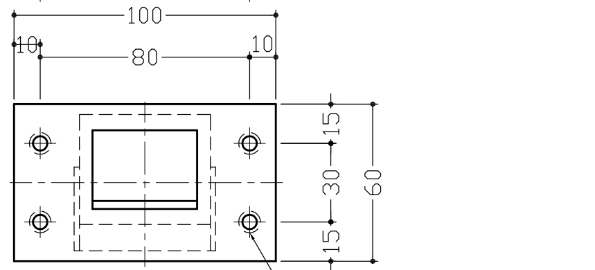
5500-3 4-5.5φ×8.3φ 皿ビス M5×12(D-8) 4本付属
