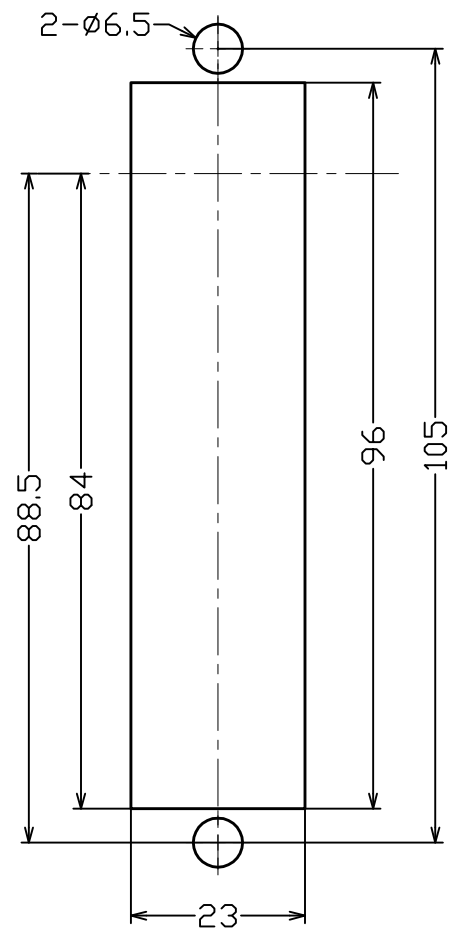
パネル切欠き寸法図
