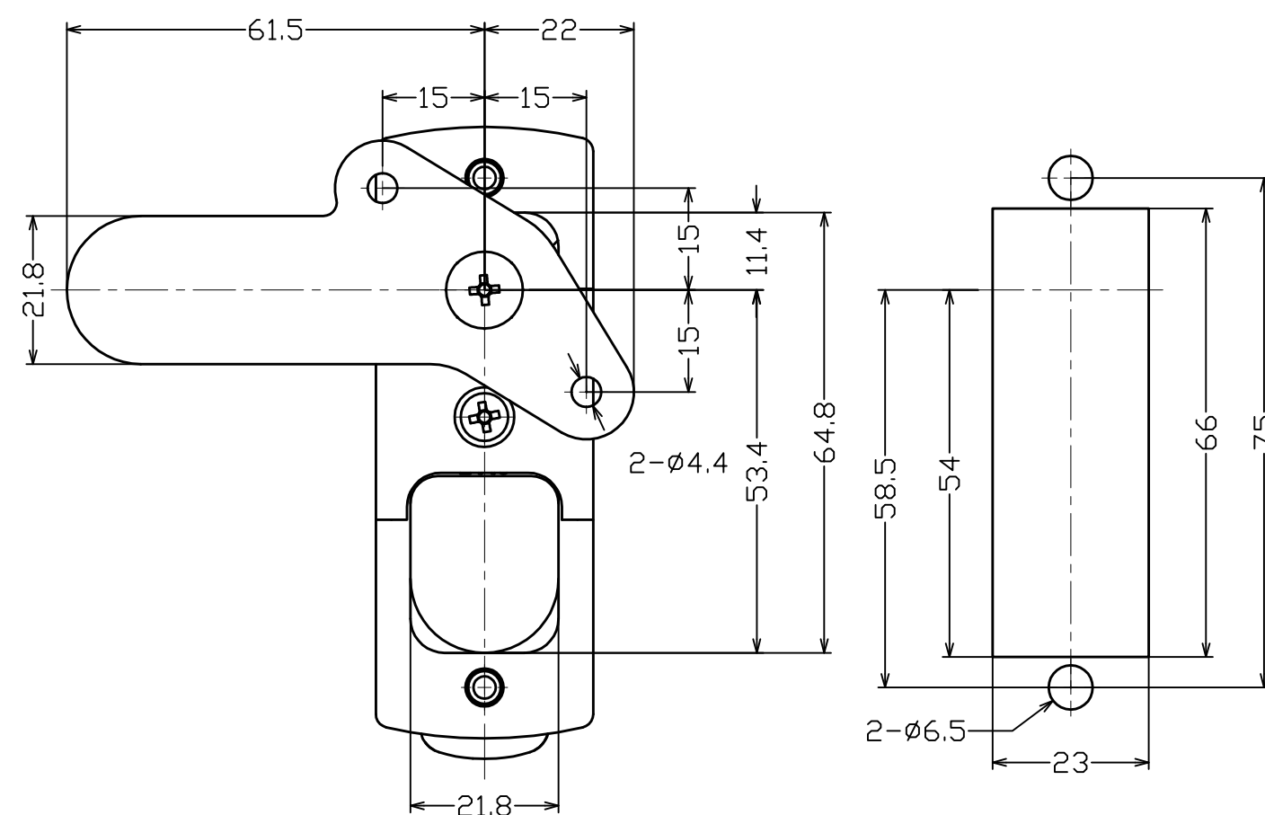
パネル切欠き寸法図
