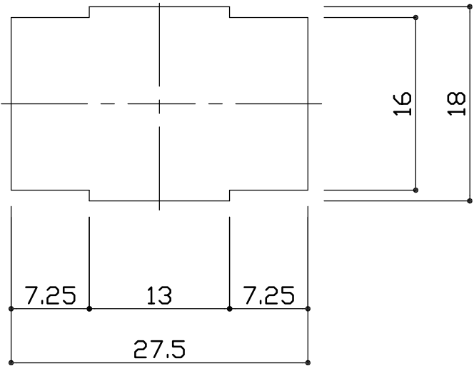
切欠き寸法
