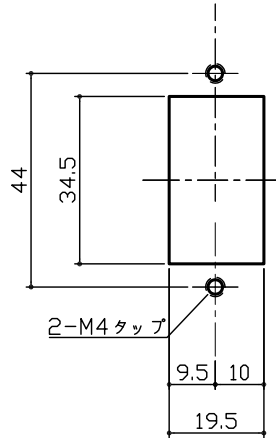
切欠き参考図
