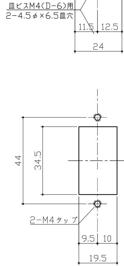
切欠き参考図
