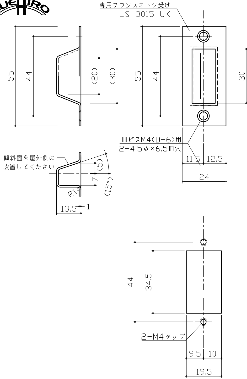
切欠き参考図
