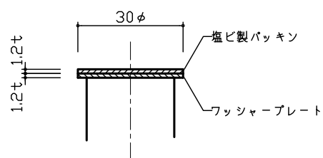
A部詳細 S=1:1
