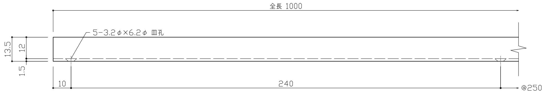
U-11(U型アルミレール) S=1:1
