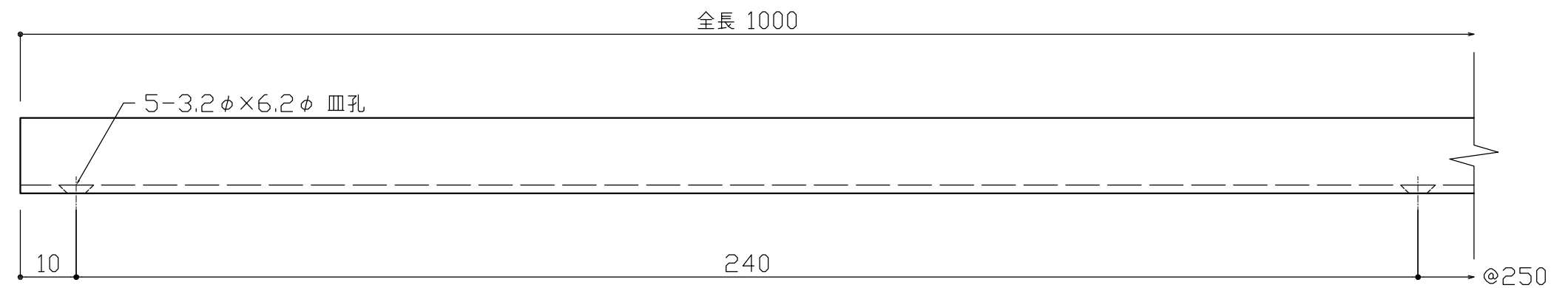
U-18(U型アルミレール) S=1:1
